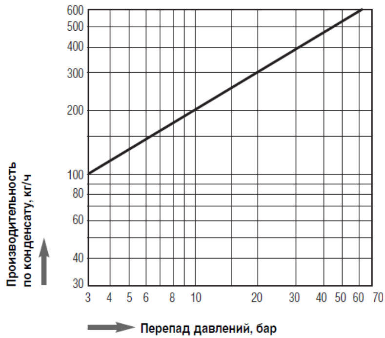
График производительности
